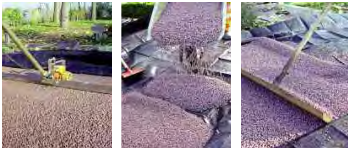
Anwendung ROMPOX-Profi Deko | Application ROMPOX-Profi Deko | utilizzo di Rompox Profi Deko
