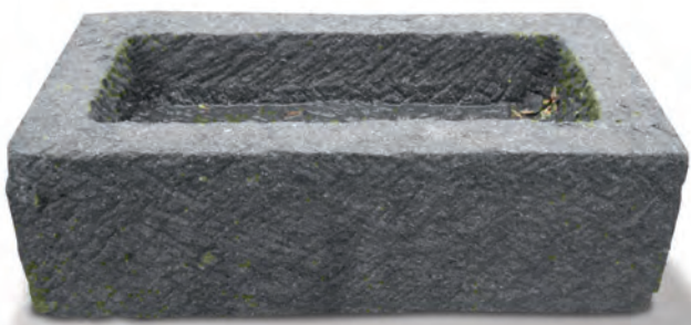
TROG BASALT RECHTECKIG Jardinière rectangulaire en basalte | Vasca rettangolare bearbeitet mit Antik Look roche volcanique brute de finition à l'aspect antique roccia vulcanica lavorata antica Art.-Nr. 300532 | 100 x 45 x H50 cm | 220 kg/Stk pce pz 300533 | 145 x 45 x H30 cm | 360 kg/Stk pce pz
