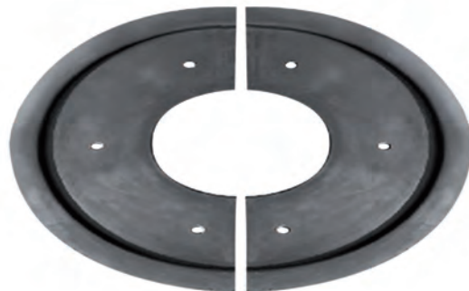
ABDECKPLATTE 140 | Couverture 140 | Copertina 140 Art.-Nr. 100160 | passend für Rundbecken 140, 2-teilig nur verwendbar mit Schwerlastensockel 52 adaptée au bassin circulaire 140, en 2 parties utilisable uniquement avec un socle pour lourde charge 52 Adatto alla vasca circolare 140 in 2 pezzi utilizzabile solo con base/zoccolo pesante 52
